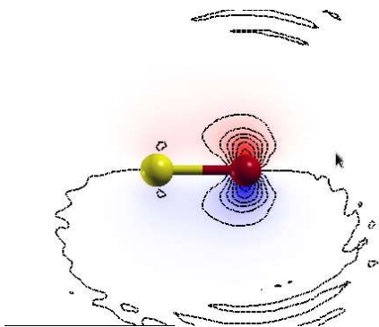
1π orbital (QE)
